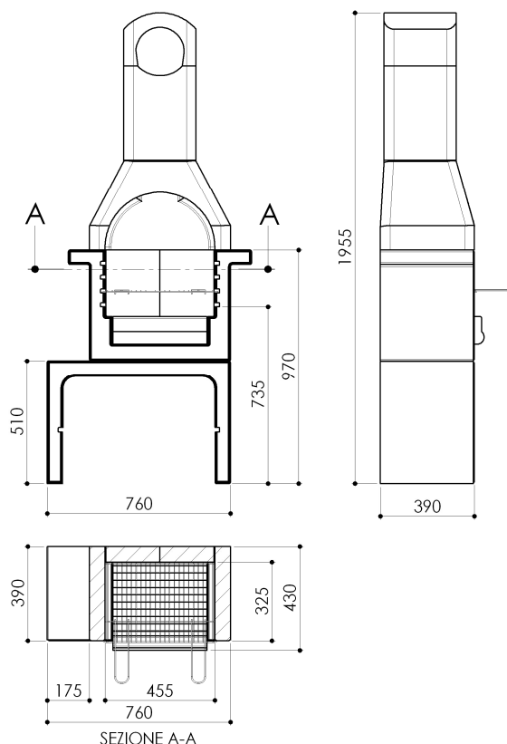
SEZIONE A-A
